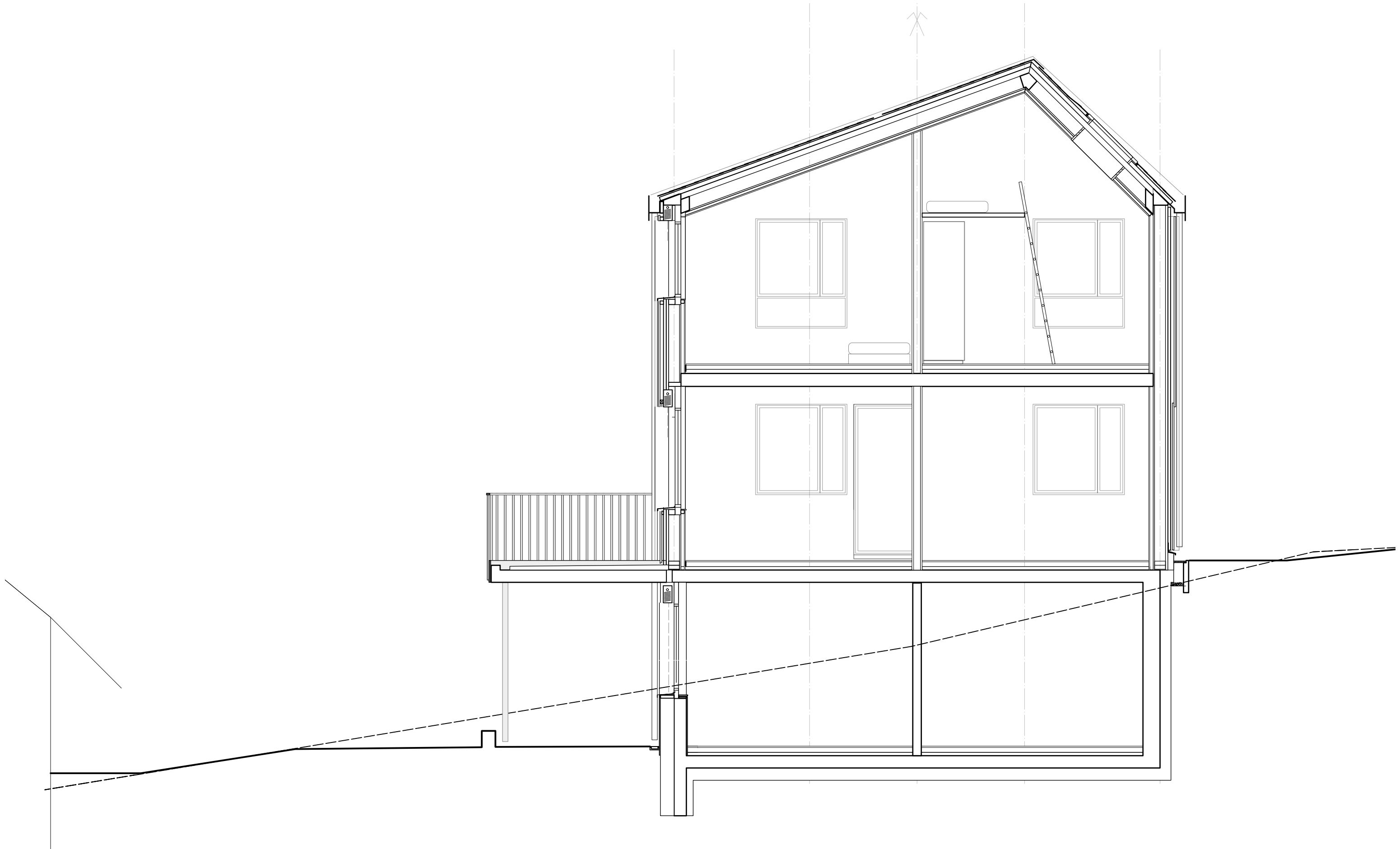
Querschnitt
