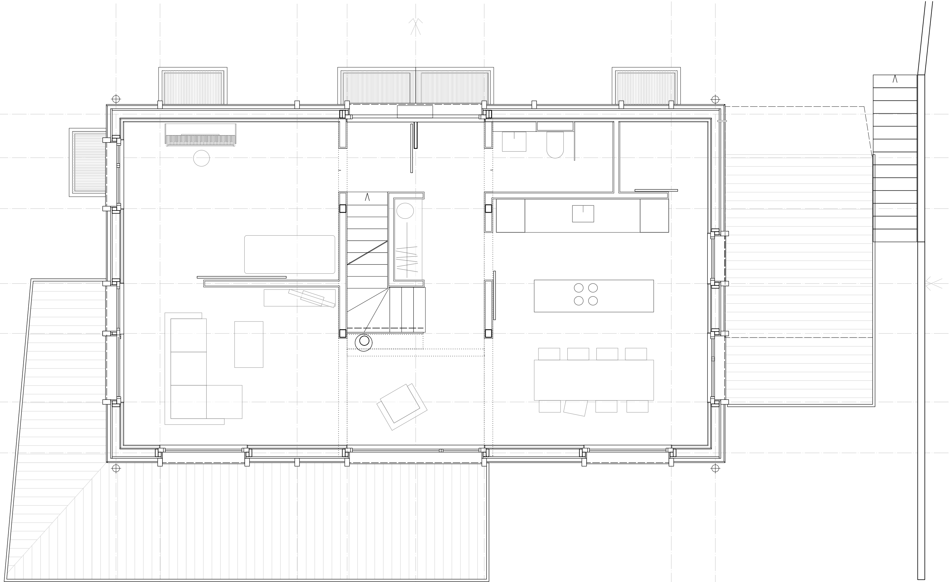
Erdgeschoss
